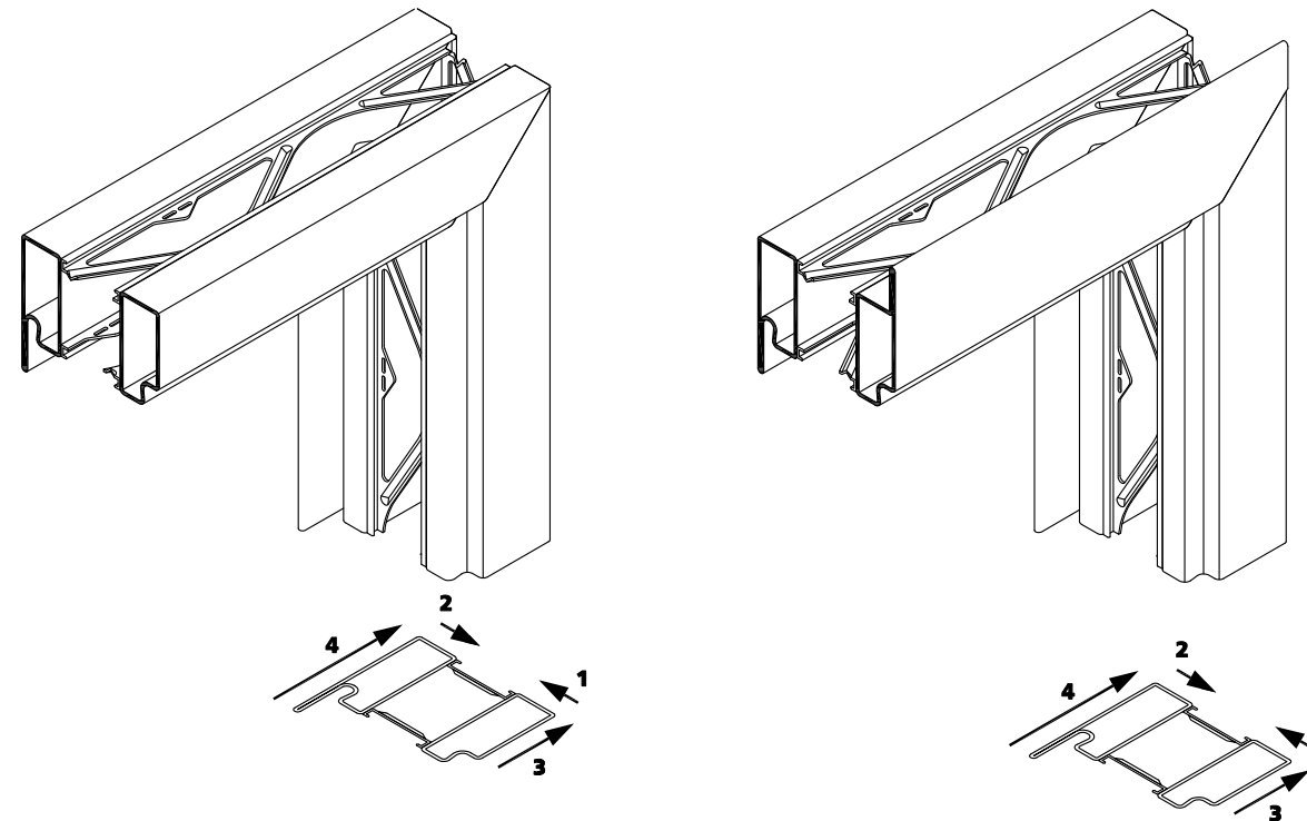
Sentido de la soldadura
