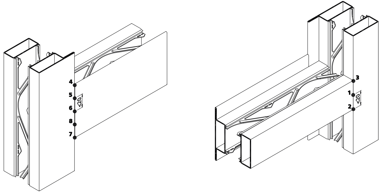
Puntos de soldadura
