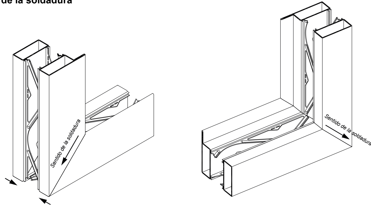
Sentido de la soldadura
