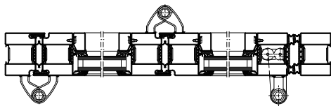
B-B Variante Perfil 50 mm
