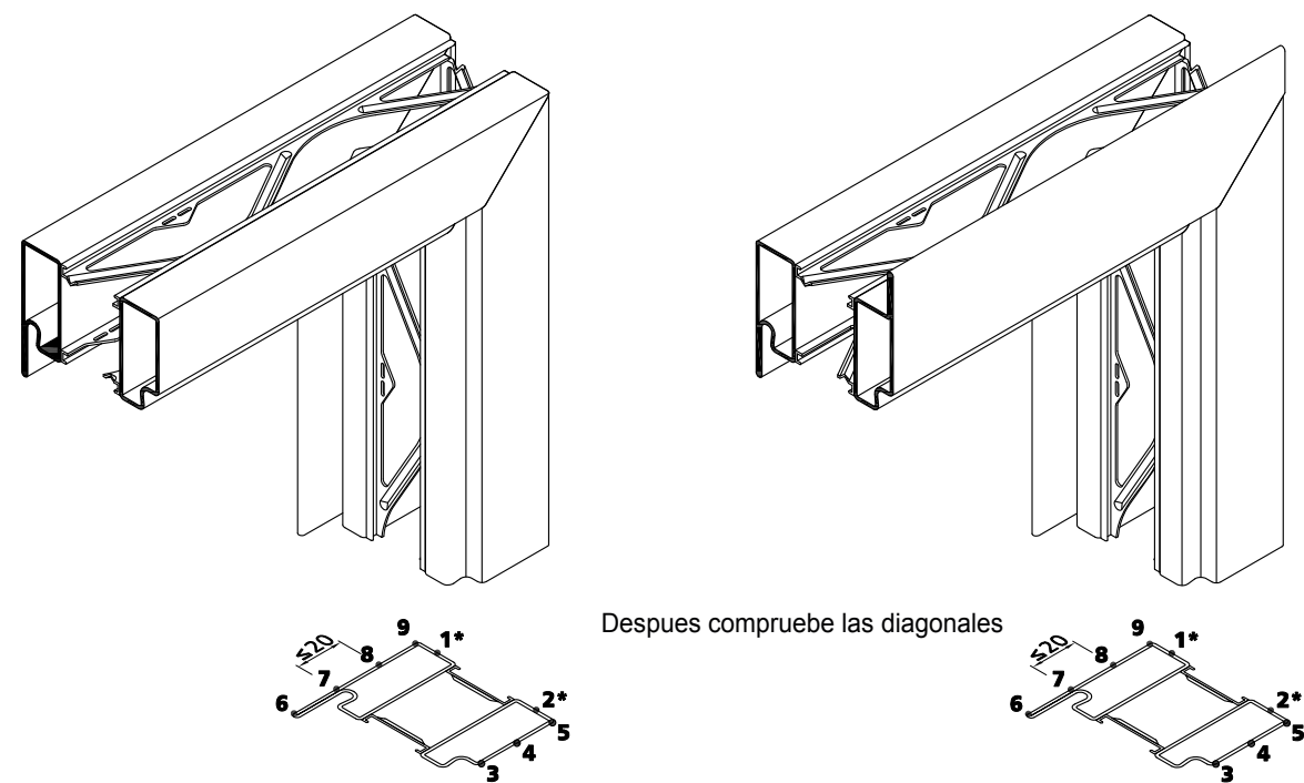
Puntos de soldadura
