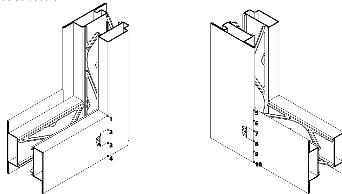
Puntos de soldadura
