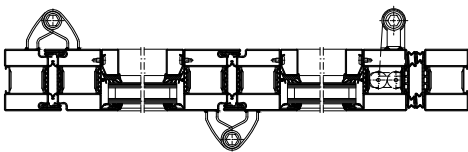
B-B Perfil Unico 50 mm
