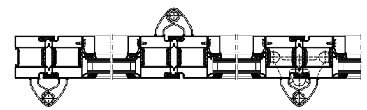
B-B Perfil Unico 50 mm
