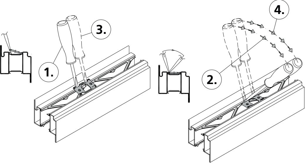
Fijación del guía 987072 (paquete de 10 piezas)
