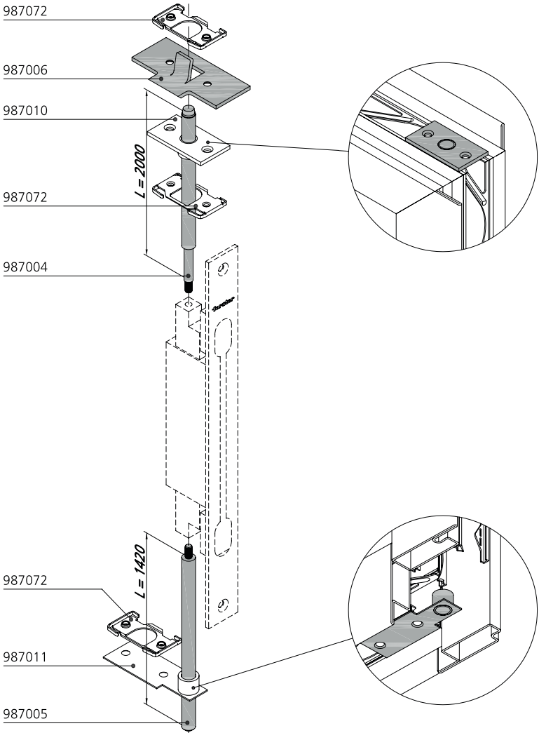
Fijación del guía 987072 (paquete de 10 piezas)
