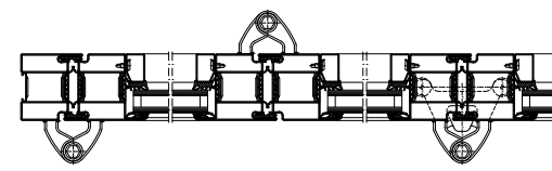
B-B Perfil Unico 50 mm
