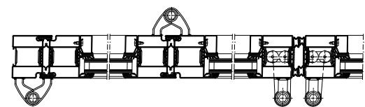
B-B Perfil Unico 50 mm
