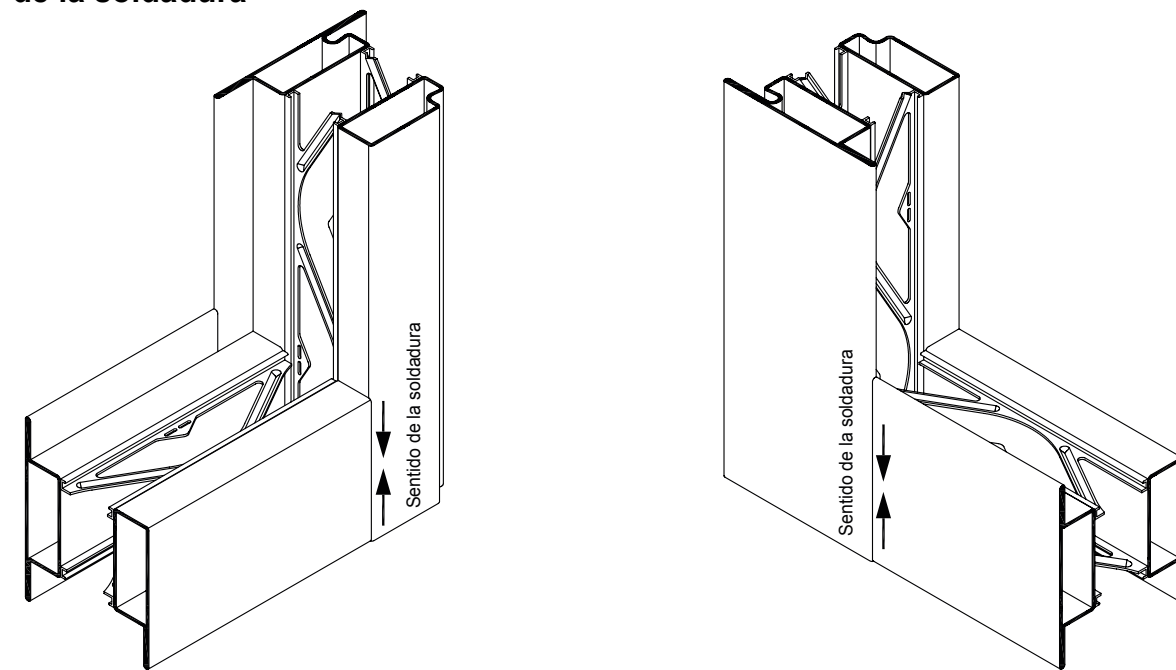
Sentido de la soldadura
